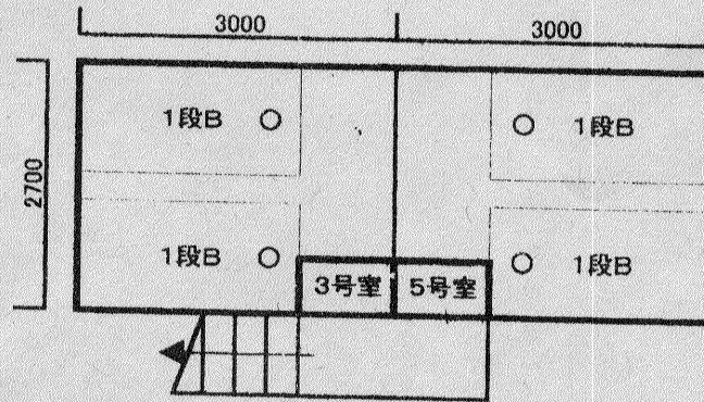
2階 平面図
